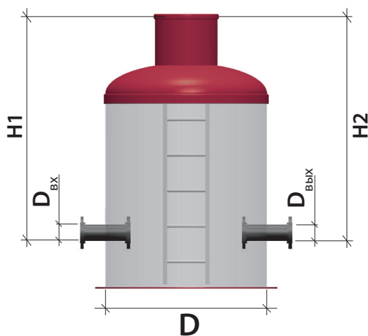
Вертикальное исполнение
